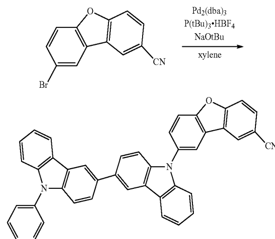
H13
