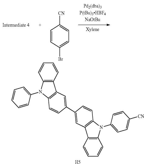
H5
