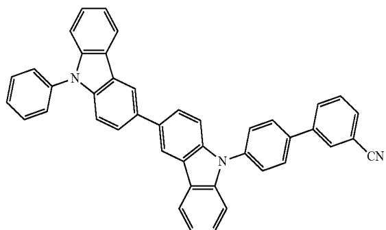
Compound F1
