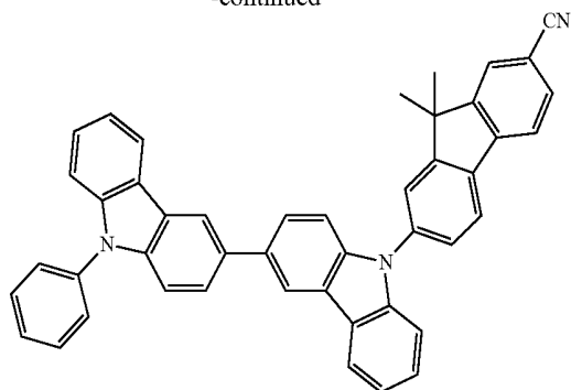
H14
