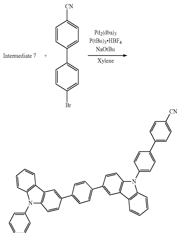
H10
