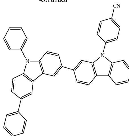
H16
