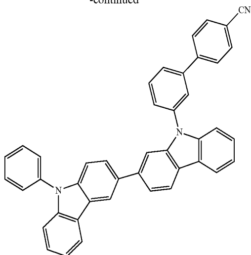
H4
