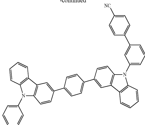
H11
